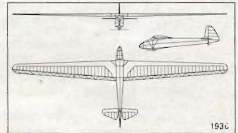
Fig 26. The 16m Mu-13 Atalante.
