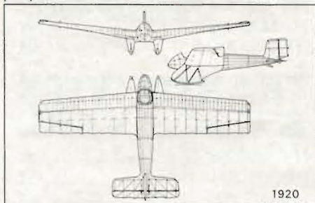
Fig 1. The 9.3m span Schwarze Teufel FVA-1 of 1920.
